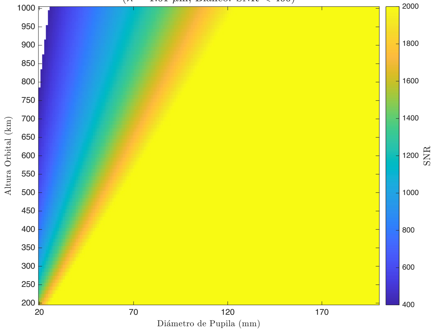
SNR - Korsch - Detector 3 ( \lambda = 1.61 \mu\text{m} , Blanco: SNR < 400)
